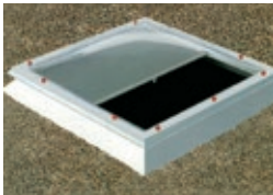
Lichtundurchlässiger Rollvorhang aus Fiberglasgewebe Farbe: Hellgrau mit alupigmentiertem Polyvinylacetat auf der Rückseite beschichtet Lichttransmissionsgrad ~ 0%
