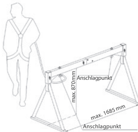
Prinzipskizze: JET-SAFETY-SET, 4-teilige Ausführung mit Anbindung an Anschlagpunkt
