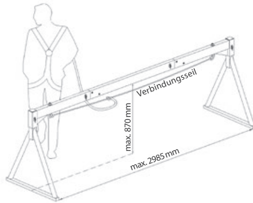
Prinzipskizze: JET-SAFETY-SET, 5-teilige Ausführung mit Verbindungsseil zwischen den Anschlagpunkten
