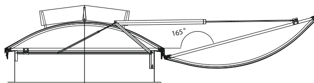
Schnitt durch JET-VARIO-THERM-Lichtband mit Vollklappe
