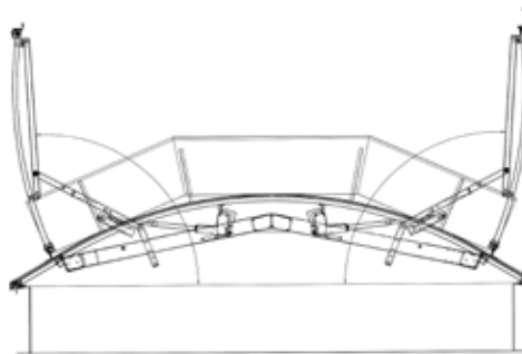
Schnitt durch JET-VARIO-THERM-Doppelklappe
